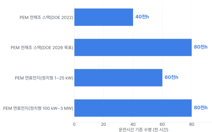
[그림 4] 스택 운전시간 기준 수명(천 시간): PEM 전해조(DOE 2022 현황·2026 목표), 정지형 PEM 연료전지(DOE 목표)
