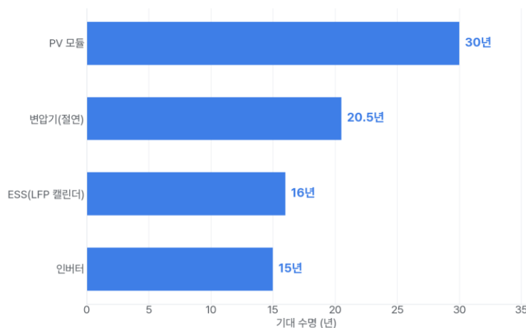
[그림 3] 설비별 기대수명(년): PV 모듈(NREL ATB 2024), 변압기 절연(IEEE C57.91), ESS LFP 캘린더(PNNL 2022), 인버터(BFH 2022)
